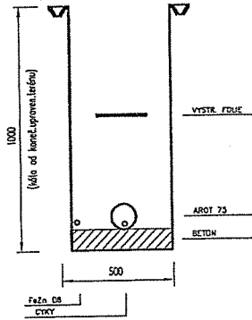
VZOROVÝ ŘEZ ULOŽENÍ ZPEVNĚNÉ PLOCHY
