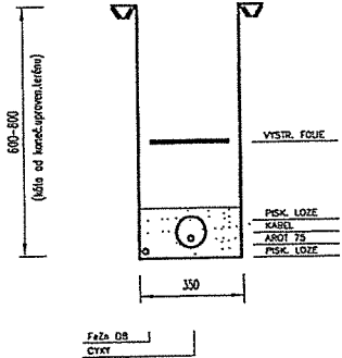
VZOROVÝ ŘEZ ULOŽENÍ VOLNÝ TERÉNEM (SOUBĚH)
